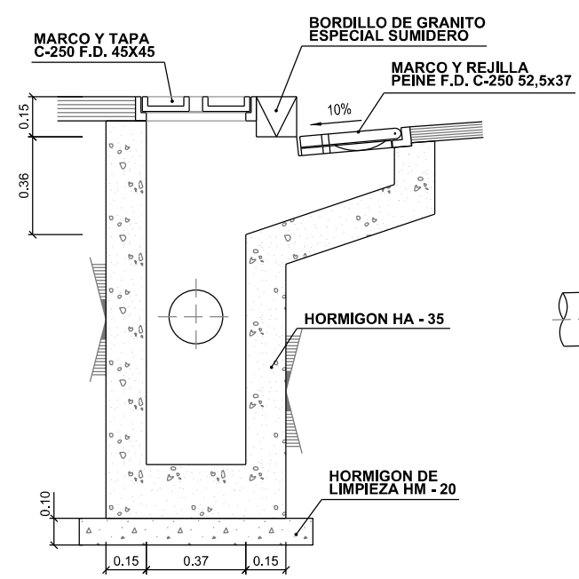
SECCION A - A
