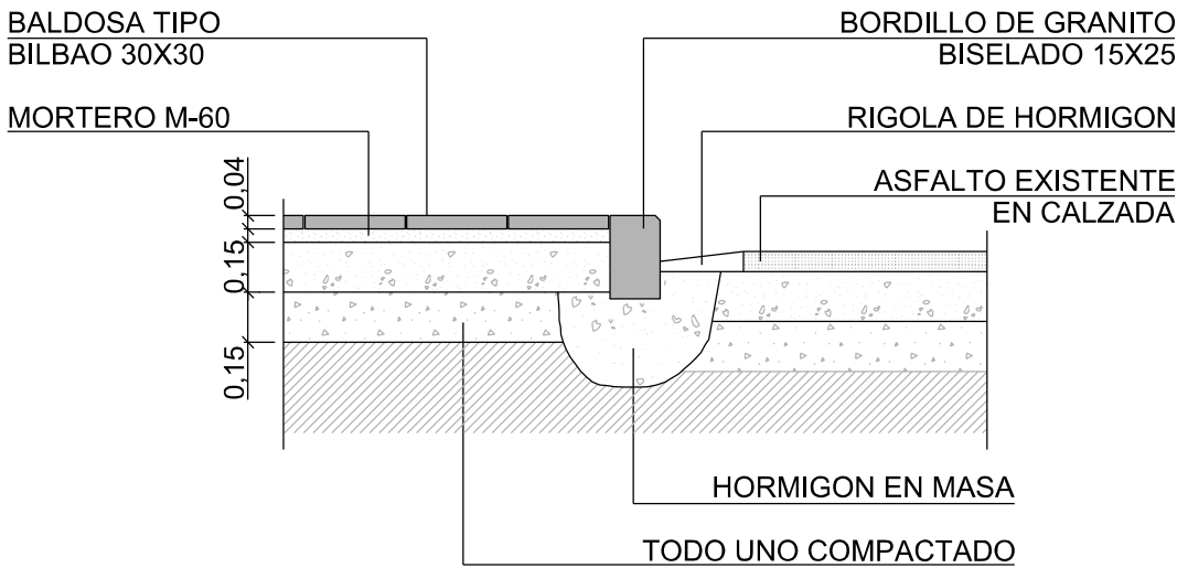
ENCUENTRO DE ACERA Y CALZADA
