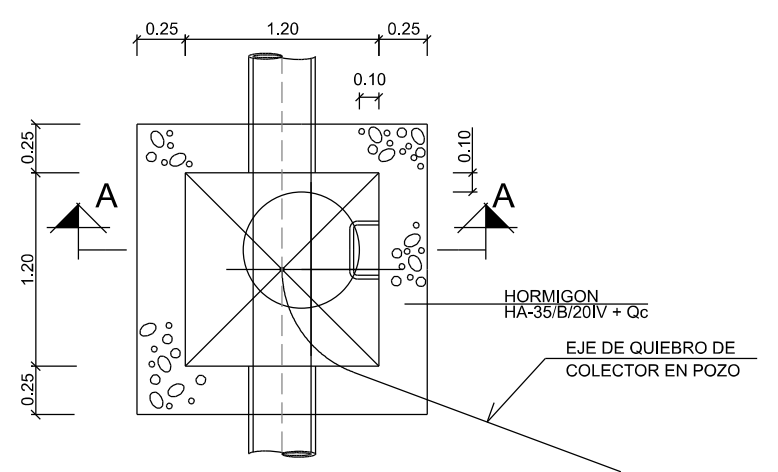
ARQUETA 1.75 < H ≤ 3.50
