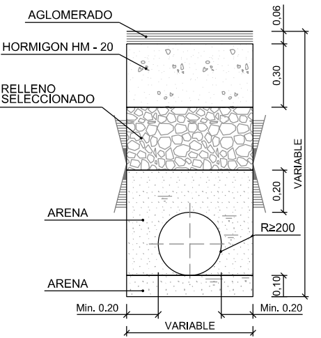
SECCION DE ZANJA EN CALZADA ESCALA 1:25
