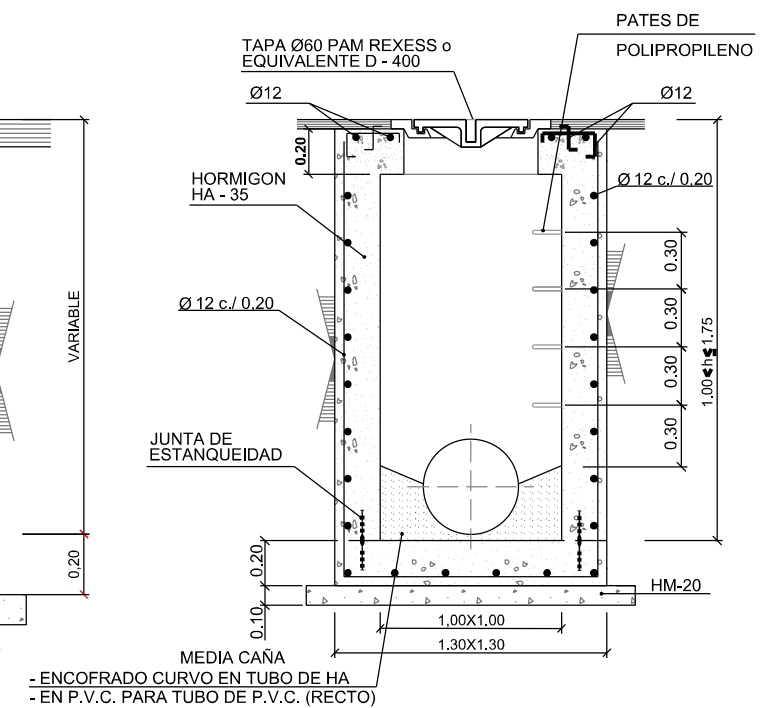
ARQUETA 1.00 < H ≤ 1.75 ESCALA 1:25
