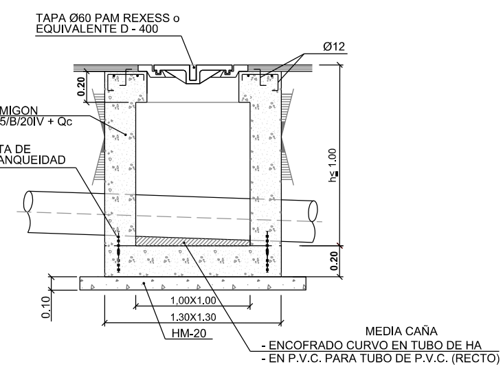
ARQUETA H < 1,00 M ESCALA 1:25
