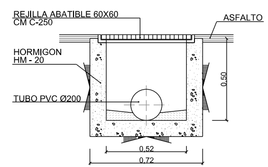
SECCION DE SUMIDERO EN ARQUETA ESCALA 1:20
