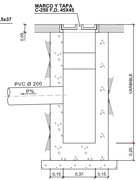
SECCION B - B
