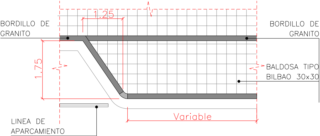
DETALLE DE FORMACION DE AVANCE DE CONTENEDORES
