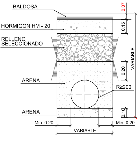
SECCION DE ZANJA EN ACERA ESCALA 1:25
