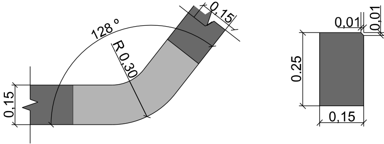
DETALLE ESQUINA BORDILLO GRANITO
