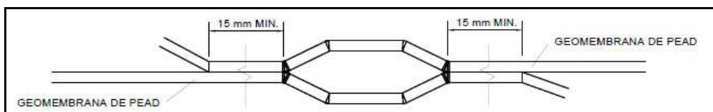
Figura 1. Soldadura por termofusión
