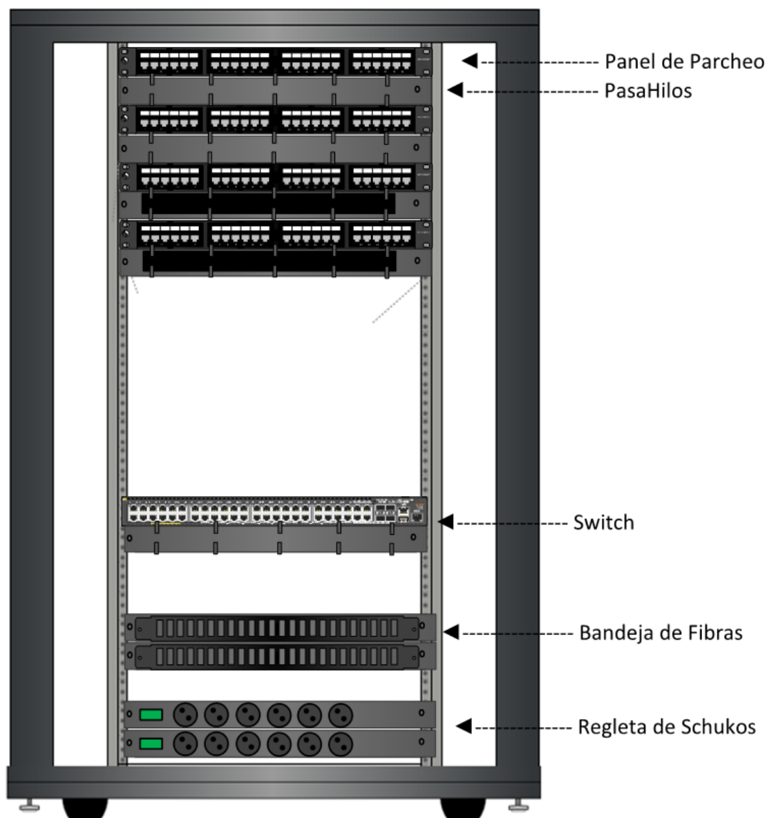
Ilustración 3: Ejemplo 1 Alzado Rack comunicaciones
