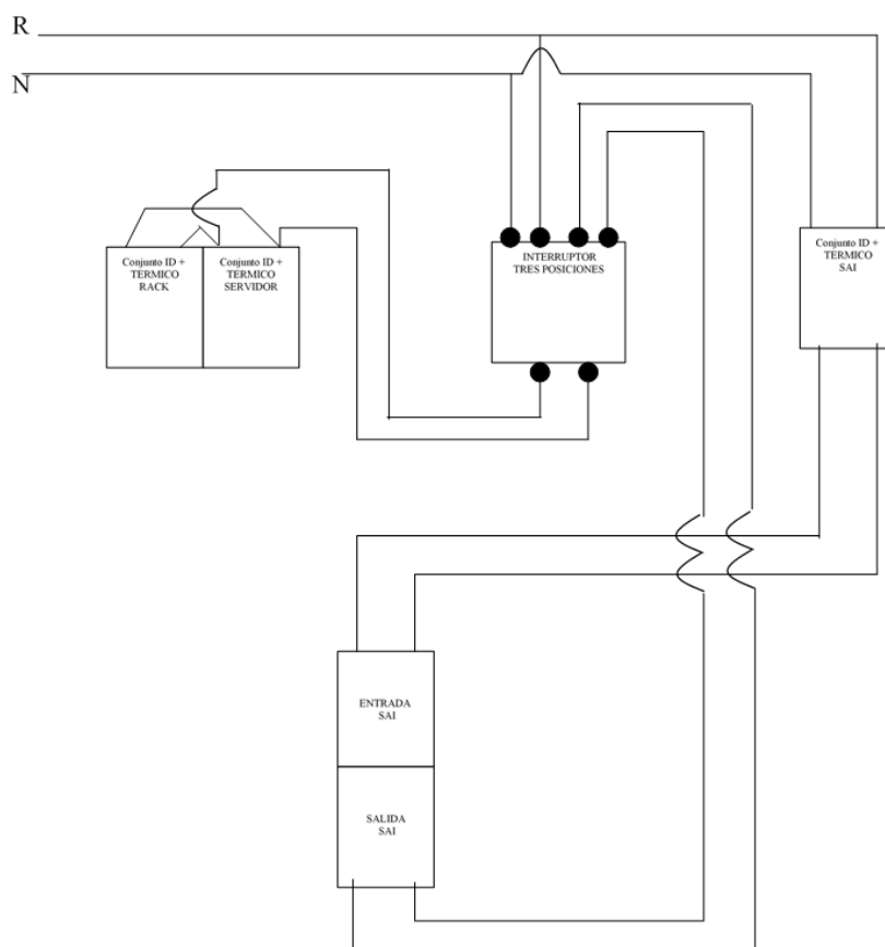
Ilustración 1 - Esquema conexonado bypass de SAI
