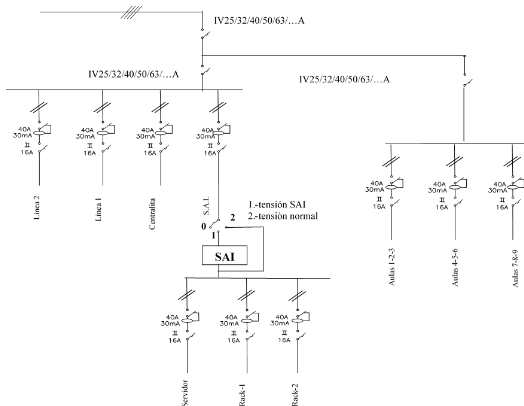
Ilustración 2: Esquema unifilar tipo (dpto. Educación)
