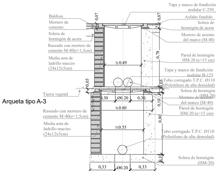
Arqueta tipo A-1
