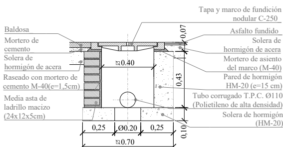
Arqueta tipo A-2
