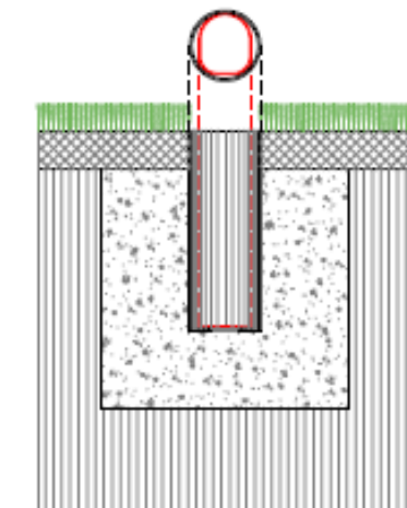
DETALLE VAINAS DE TUBO DE ACERO GALVANIZADO
