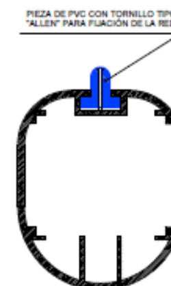
DETALLE PERFIL DE ALUMINIO POSTES Y LARGUERO
