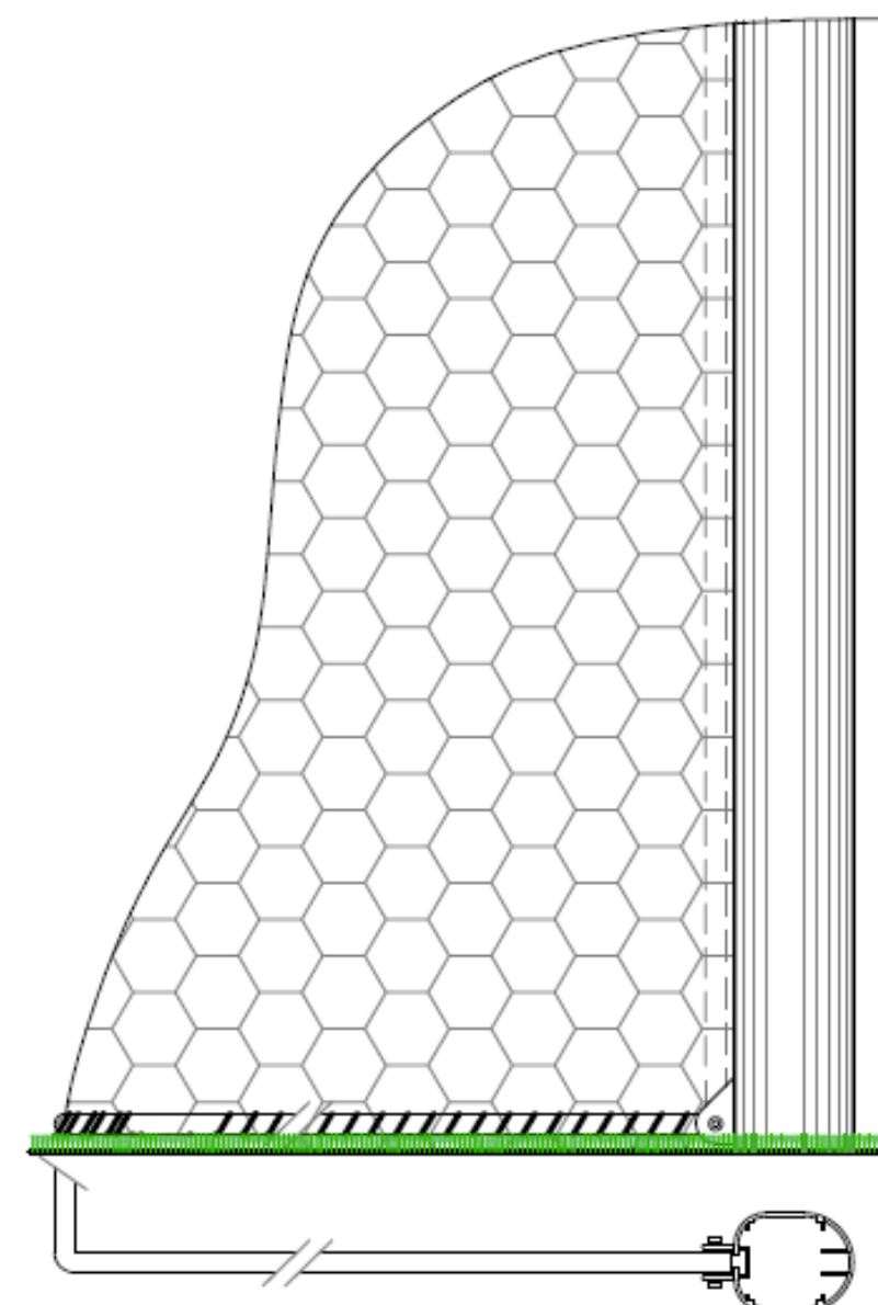
DETALLE DE LA FIJACIÓN DE LA BARRA DE ANCLAJE INFERIOR DE LAS REDES CON LOS POSTES DE LA PORTERÍA
