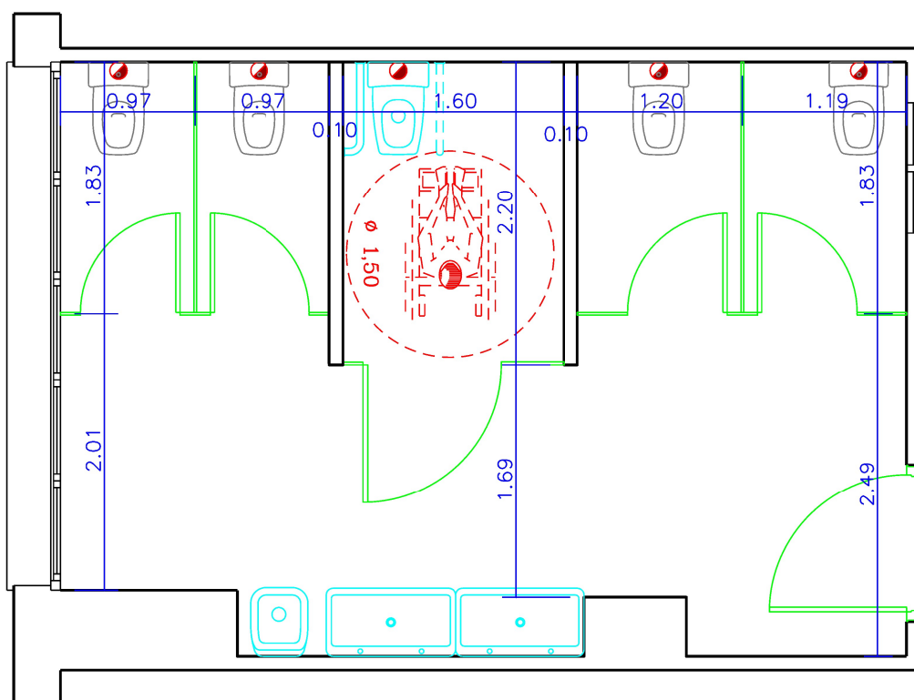
ESTADO REFORMADO Escala: 1/50
