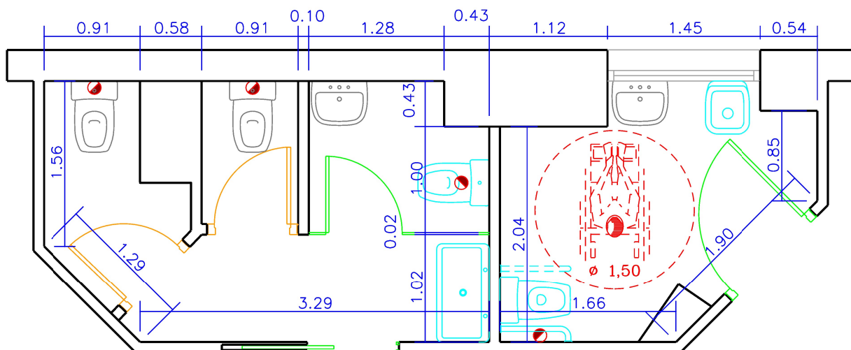
ESTADO REFORMADO Escala: 1/50
