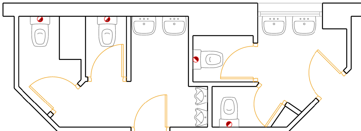
ESTADO ACTUAL Escala: 1/50
