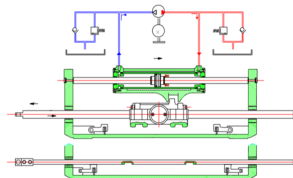
Posición intermedia del accionamiento
