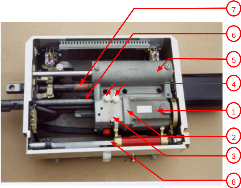
Interior del accionamiento electrohidráulico
