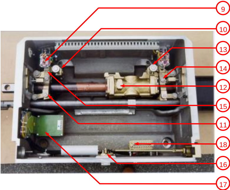
Interior del accionamiento electrohidráulico sin la unidad
