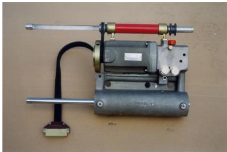
Fotografía 3: Vista de la unidad impulsora.
