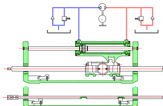
Posición final del accionamiento
