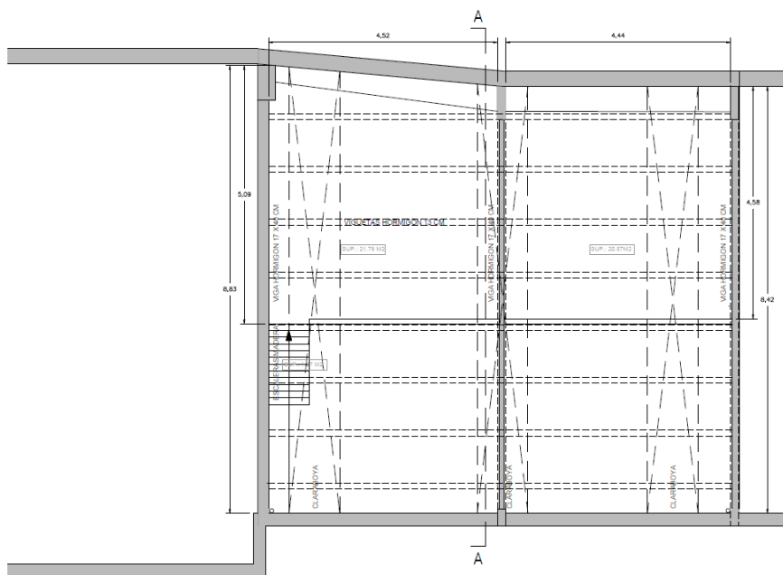
Figura 3.- Planta baja pabellón
