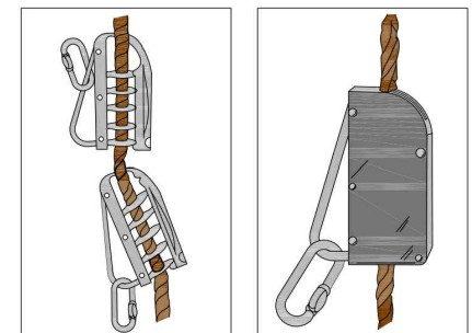
ANCLAJES CINTURON DE SEGURIDAD (Seguro automáticos anticaídas)
