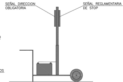
VISTA LATERAL
