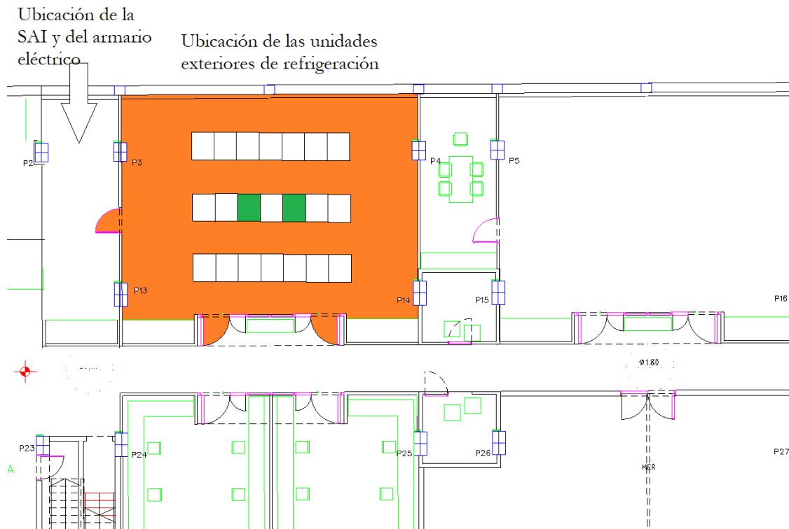
Figura 2. Distribución final de los racks del supercomputador en el CPD con las dos salas ya unidades (en naranja), ubicación del posible hueco de la SAI y armario eléctrico y ubicación de las unidades exteriores de la refrigeración.
