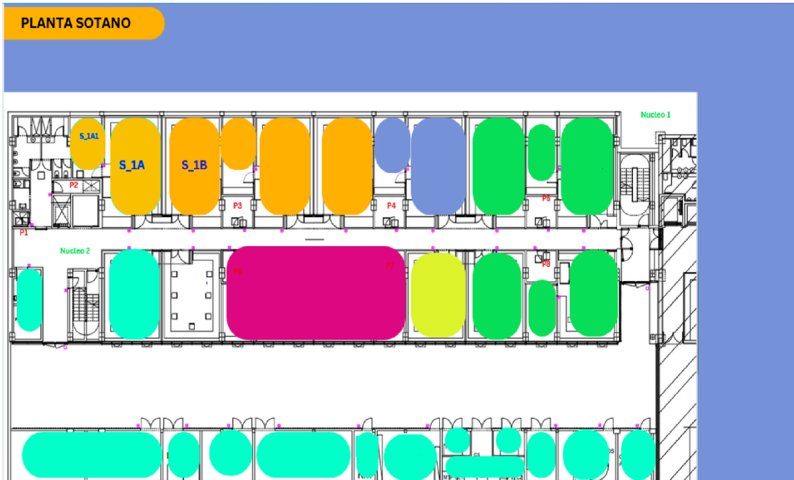
Figura 1. Planta sótano del edificio. Los racks de computación serán instalados en una unión de los huecos S_1A y S_1B (se tirará la pared que ahora los une) y la SAI y el armario eléctrico se instalarán preferiblemente en el hueco S_1A1, aunque también estarán disponibles los otros tres espacios de color naranja si fueran necesarios.
