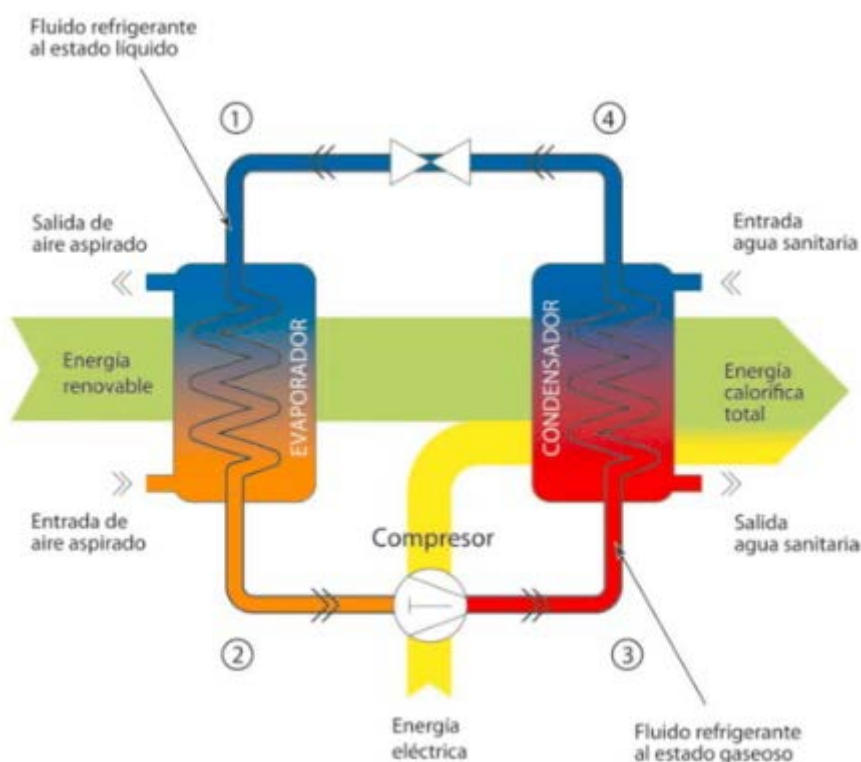
Imagen 2.- Esquema de funcionamiento de circuito frigorífico.
