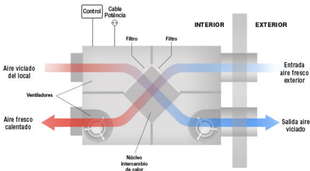
Imagen 3.- Esquema de flujos por el interior del recuperador de calor.
