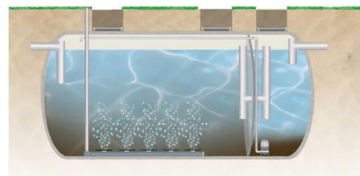
REACTOR DECANTADOR
