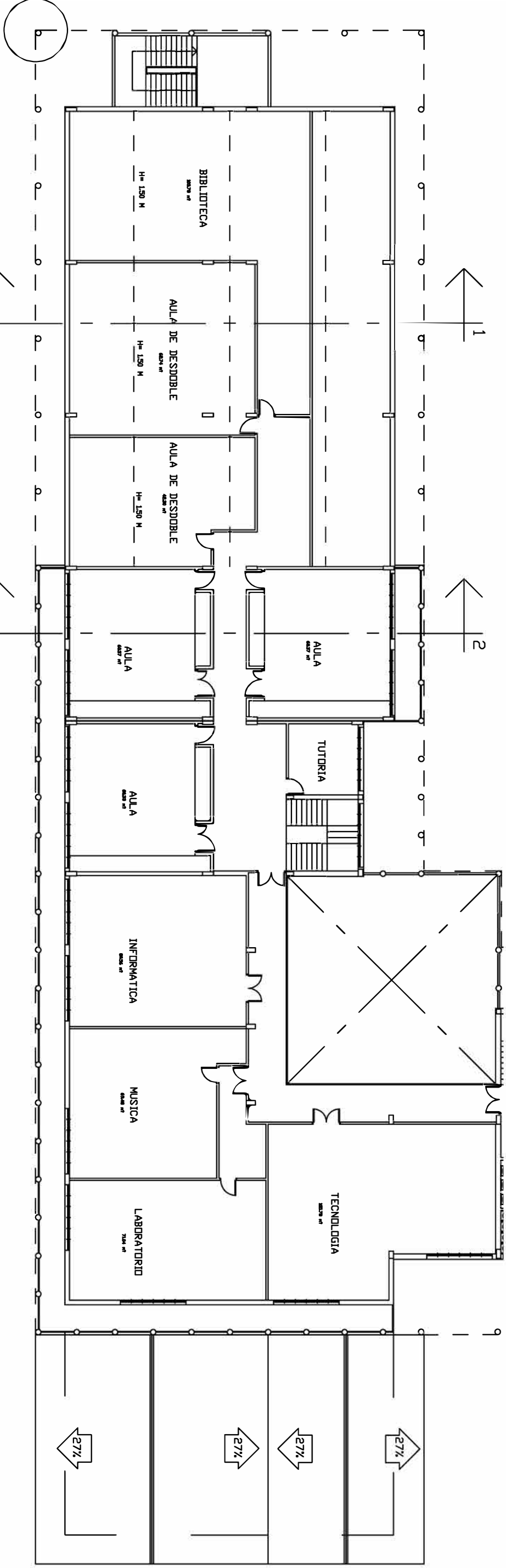
XABIER MUNIBE IKASTOLA-SEGUNDA PLANTA
