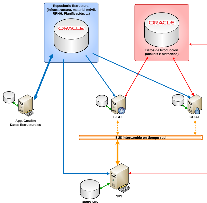
Fig. 2: Modelo de intercambios en el bus CUN
