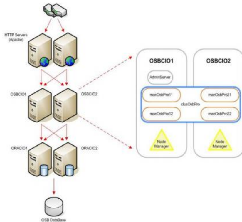
Fig. 4: Arquitectura de servidores
