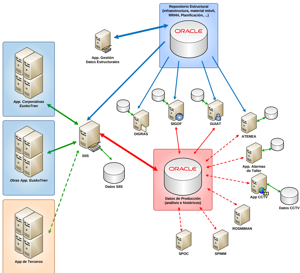
Fig. 1: Arquitectura general de la Base de Datos
