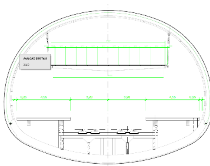
Sección tipo en Trayecto Estación
