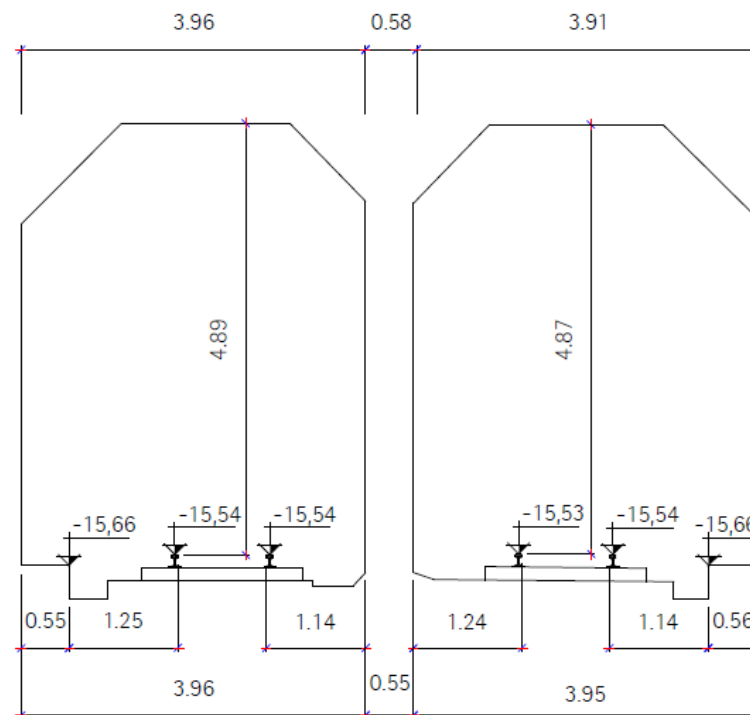
Sección tipo en Subfluvial Olabeaga
