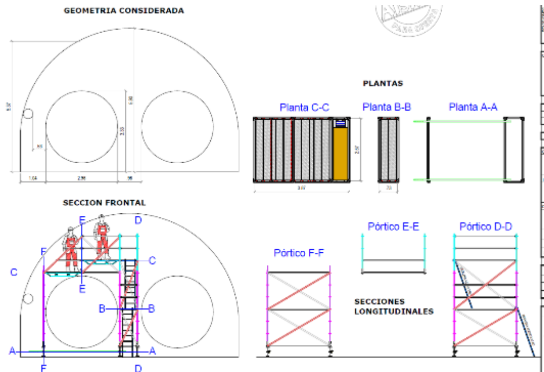
Sección tipo de caverna de ventilación
