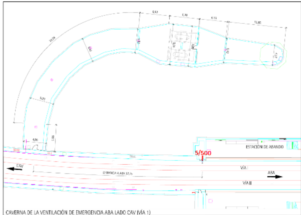
Planta cavernas de ventilación
