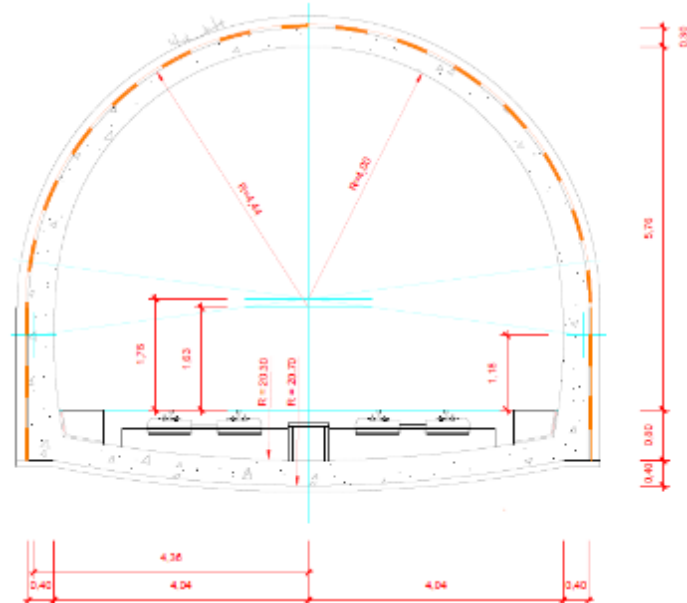
Sección tipo en Trayecto entre estaciones
