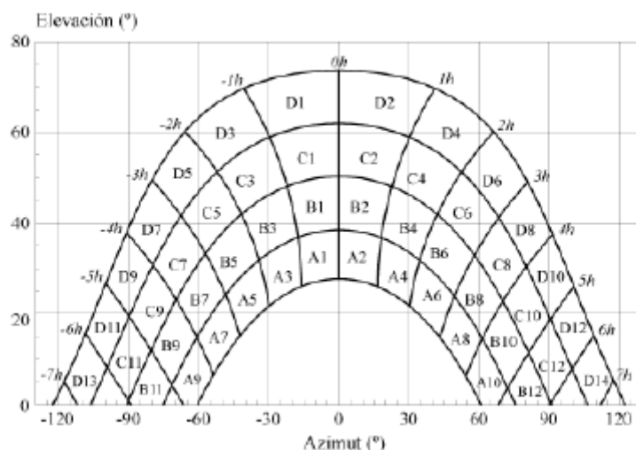
Ilustración 9 Diagrama de la trayectoria del sol
