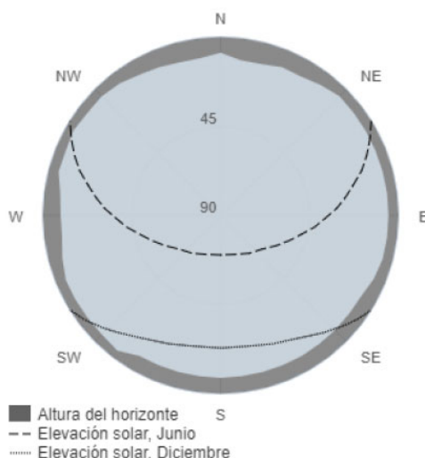
Ilustración 7 Perfil del horizonte según PVGIs en el campo de fútbol de Beasain
