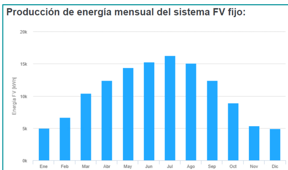
Gráfica 5 Producción de energía mensual en la cubierta del campo de fútbol con orientación al sur-este
