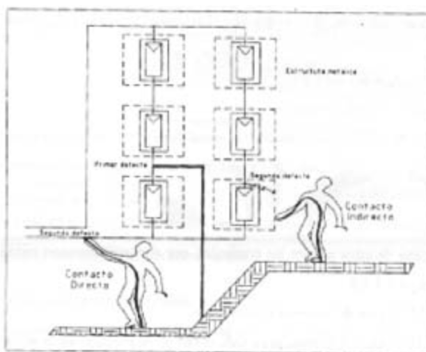
Ilustración 8 Riesgo eléctrico en un generador fotovoltaico
