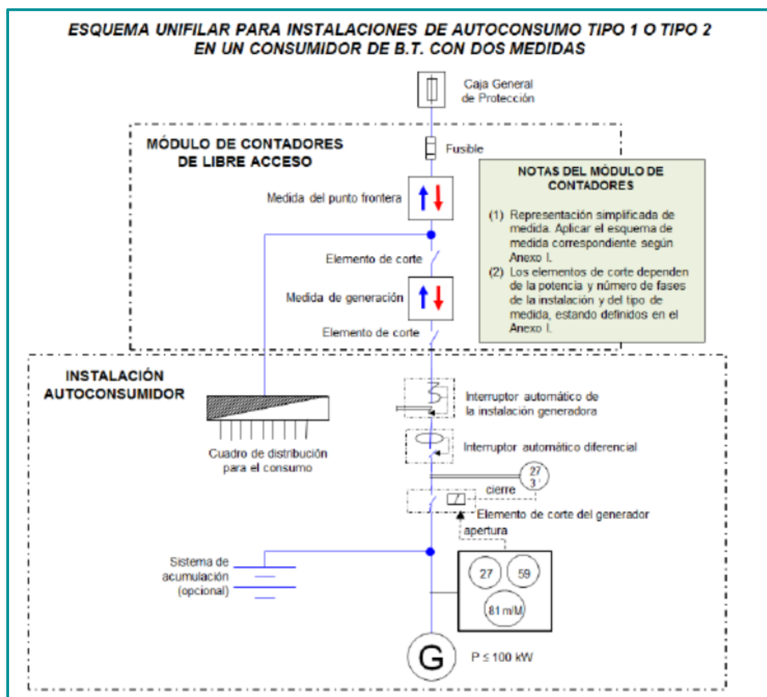
Ilustración 6 Esquema de medida (PF+PG) según la Memoria técnica de la empresa distribuidora
