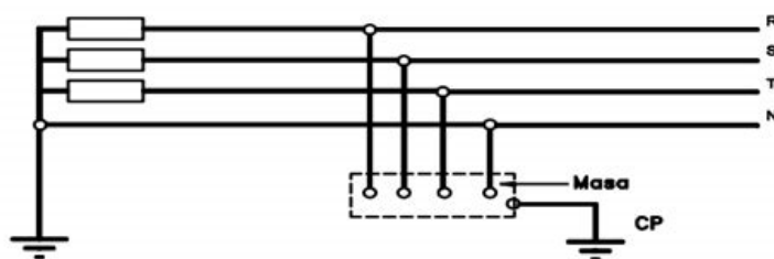
Ilustración 4 Esquema TT de conexión a tierra
