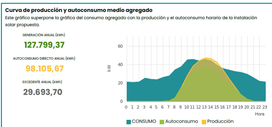
Gráfica 3 Consumo por horas y la curva de generación
