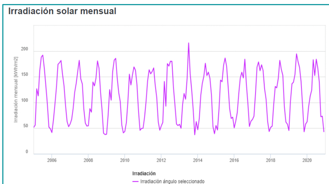
Gráfica 4 Radiación media anual sobre el tejado del CAMPO DE FÚTBOL DE BEASAIN
