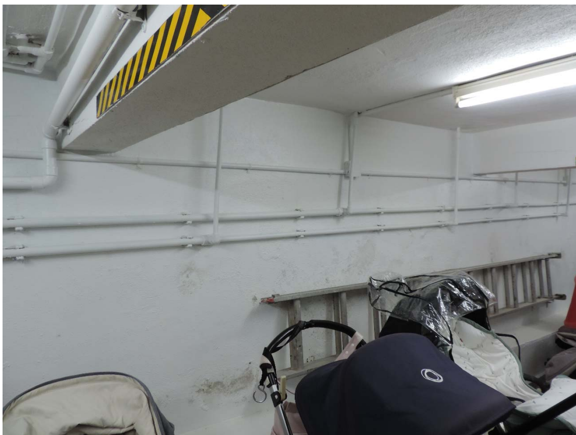
Conductos del circuito 1 de calefacción en planta baja
