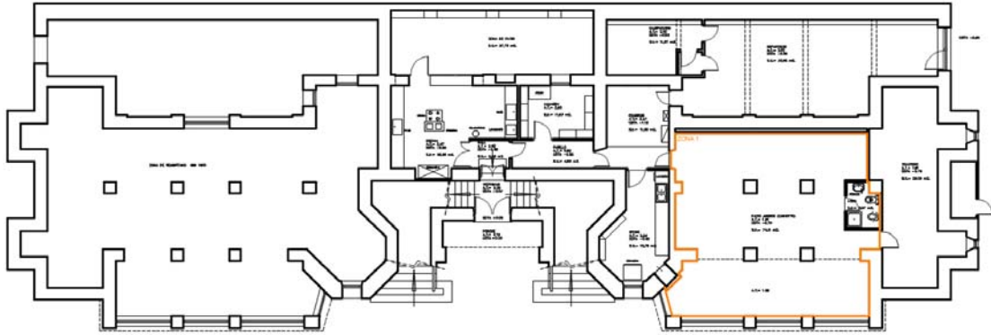
Distribucion de zona 1 de calefacción en planta baja
