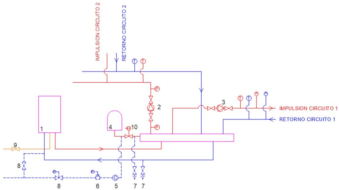
Esquema de la instalacion actual de calefaccion
