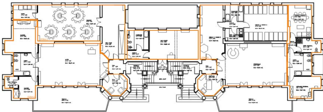
Distribucion de zonas 2-3-4-5-6 de calefacción en planta superior
