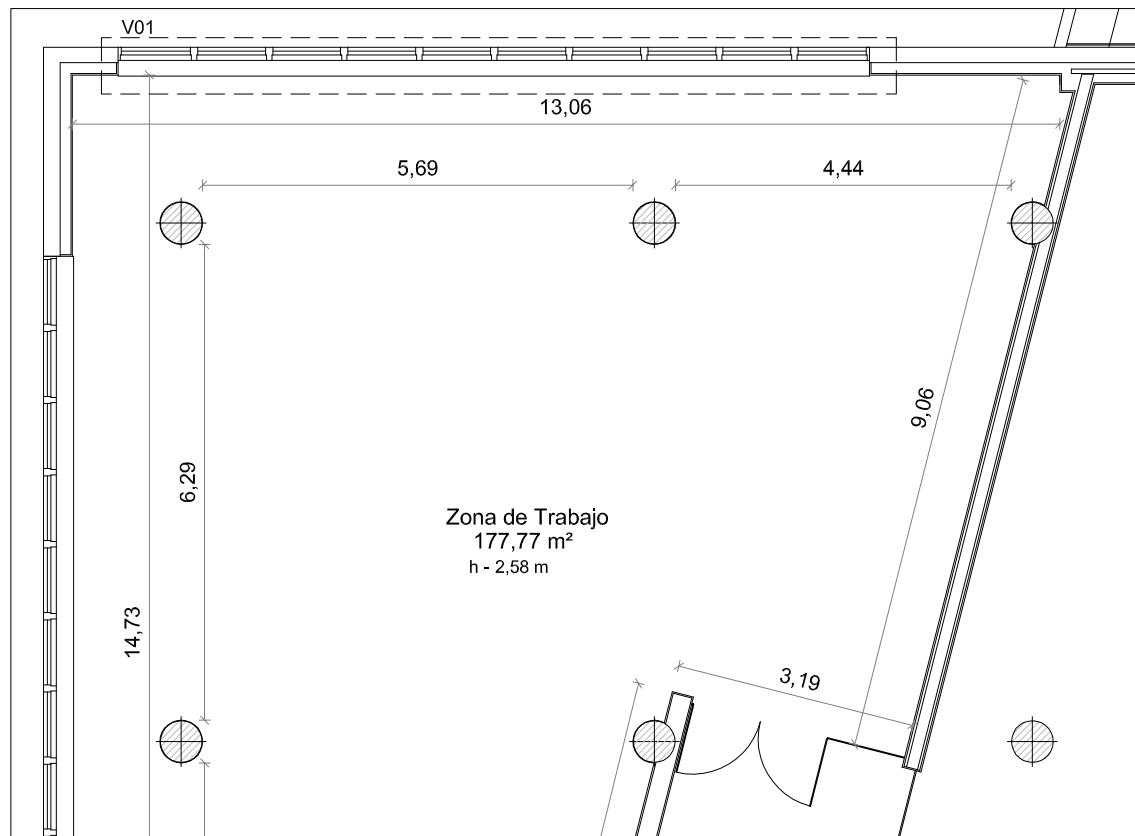
PLANTA BAJA_ESTADO ACTUAL
