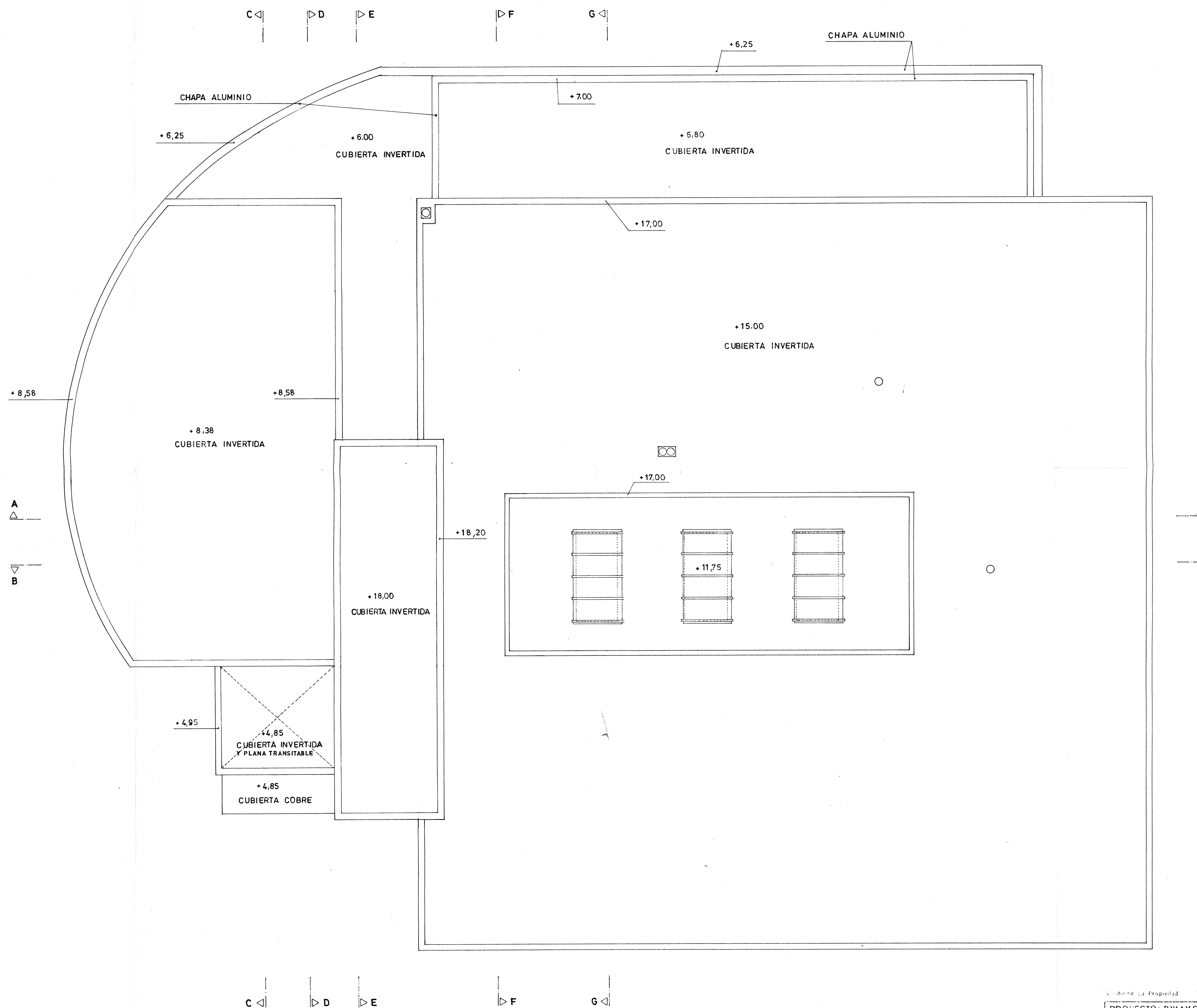
PLANTA DE CUBIERTA COTAS +15.00 y +18.00
