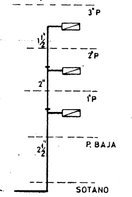
DETALLE SECC. TUB. BIE SEGUN PLANTAS
